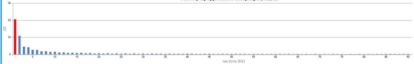
Спектр продольной вибрации, dB, Hz
